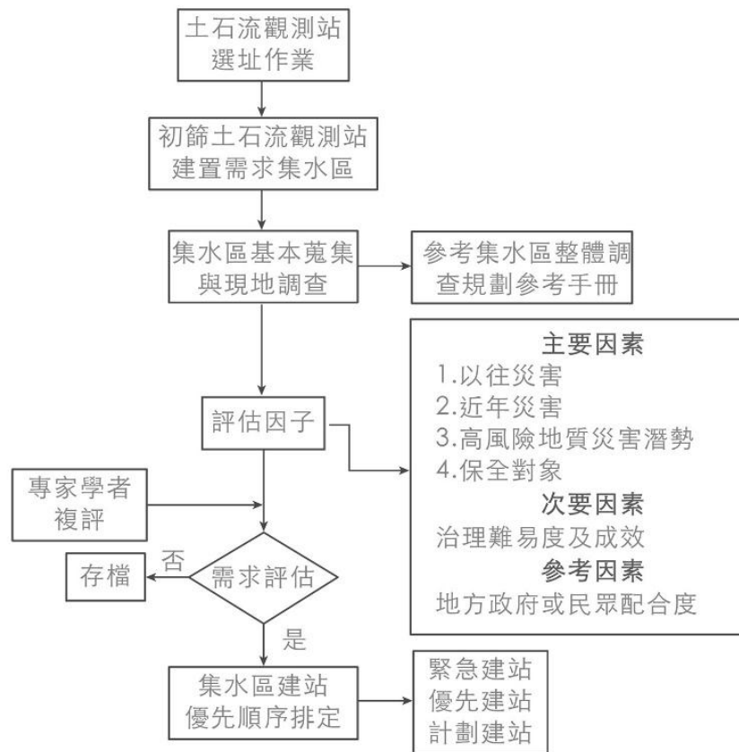
圖 6-2-4 土石流觀測站選址與評估
