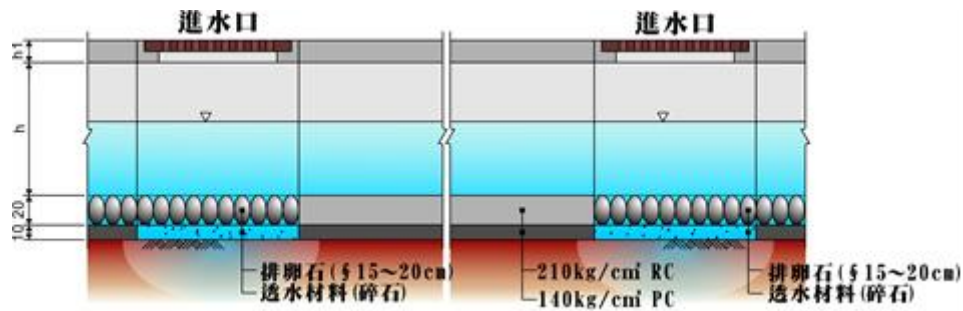
圖 3-2-8 滲透性側溝範例示意圖
