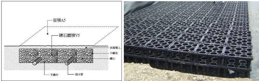
圖 5-1-8 地下礫石層與組合式蓄水框架的地下貯集滲透工法 資料來源：內政部營建署「建築基地保水設計技術規範」，108 年。
