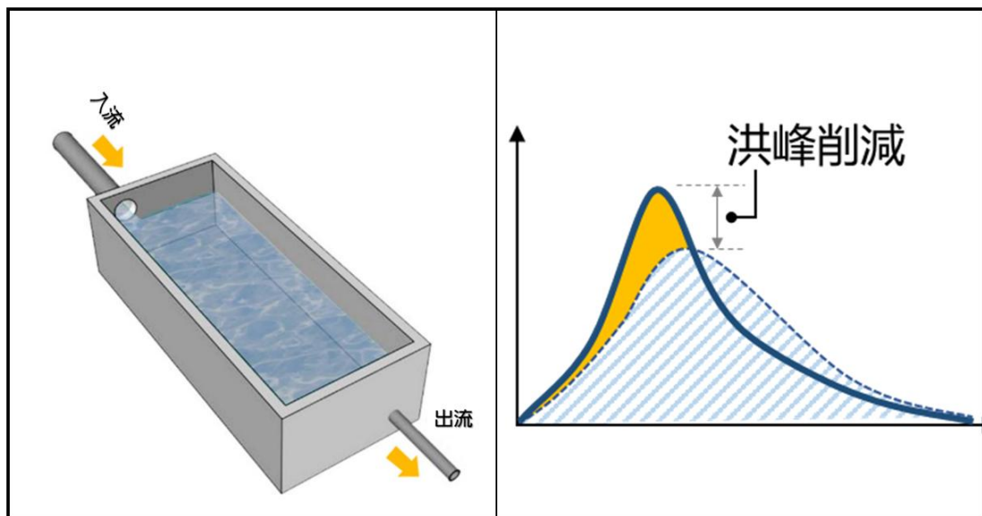
圖 5-1-16 在槽滯洪設施示意圖
