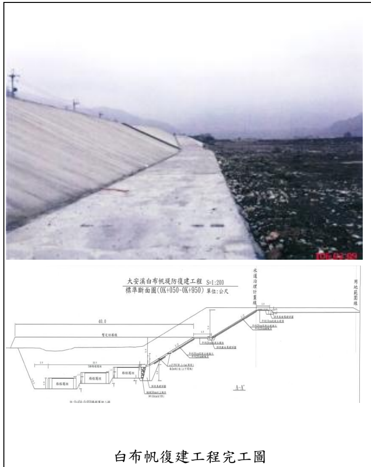
圖 6-3-2 大安溪白布帆堤防復建工程 資料來源:經濟部水利署
