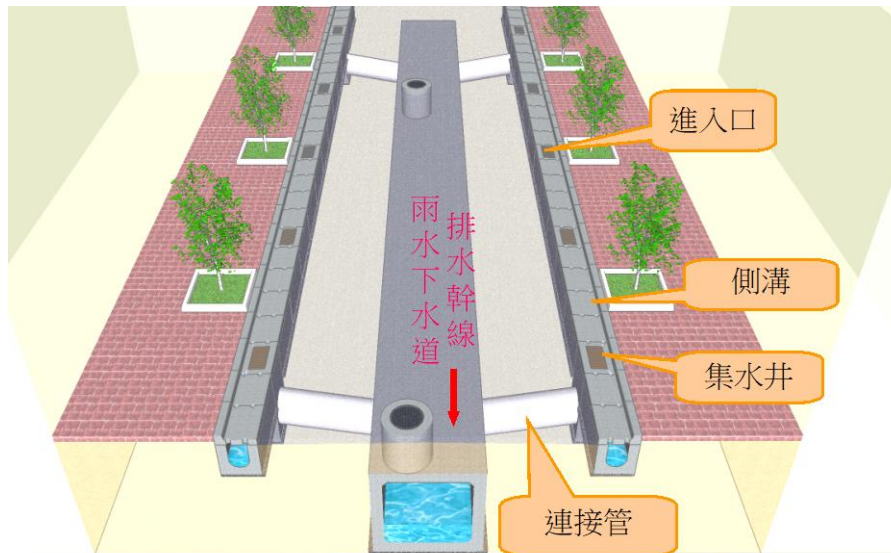
圖 3-2-5 雨水下水道及地面逕流收集系統示意圖
